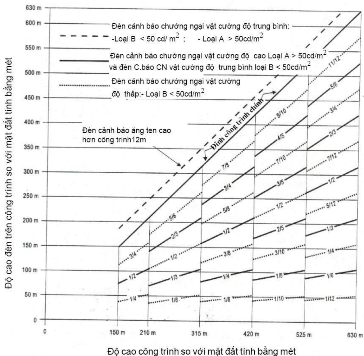
Hình A5-7. Hệ thống đèn cảnh báo CNV kép cường độ cao/ trung bình, Loại A/Loại B
