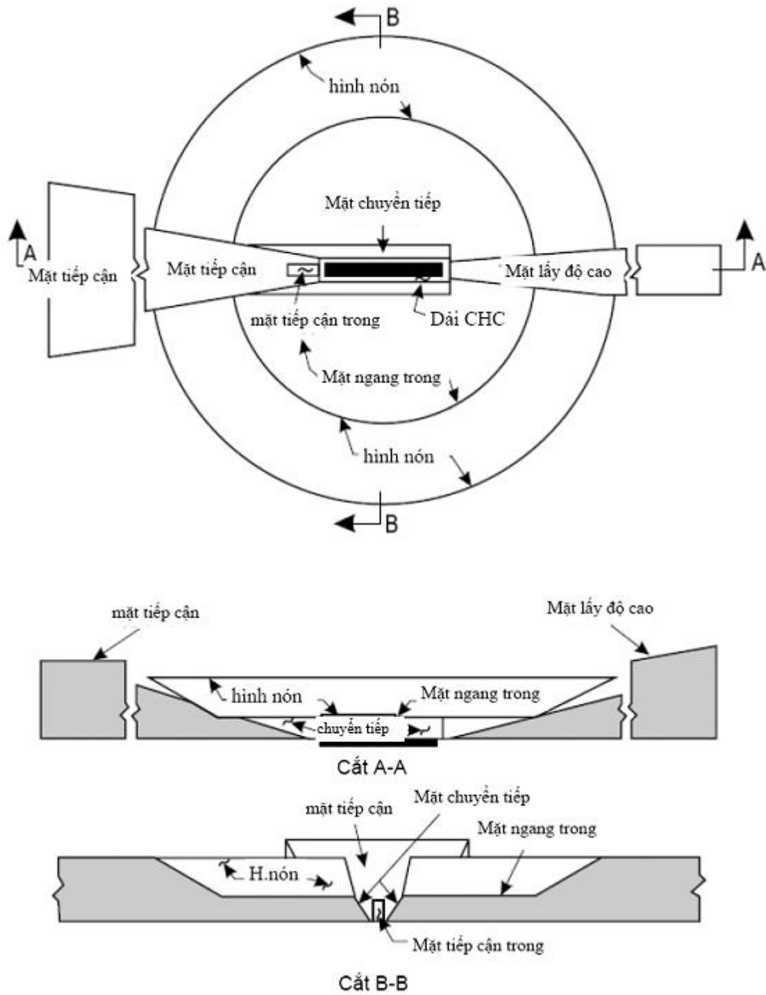
Hình 4-1. Giới hạn bề mặt tĩnh không
