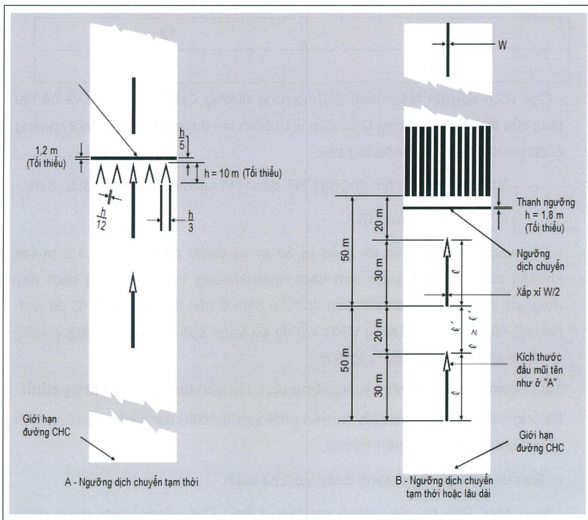
Hình 5-4. Sơn tín hiệu đánh dấu ngưỡng đường cất hạ cánh bị dịch chuyển
