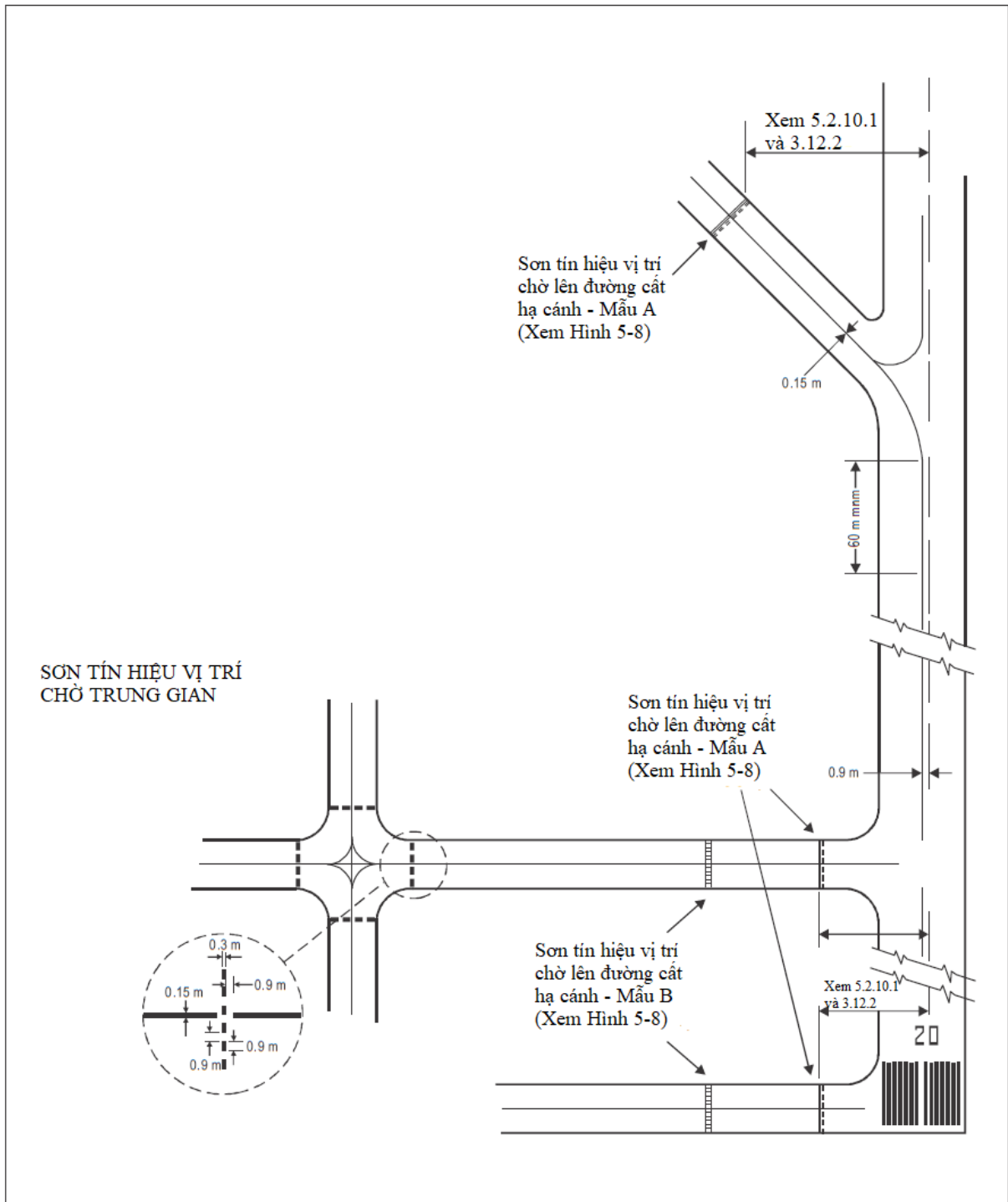
Hình 5-6. Sơn tín hiệu đường lăn (cùng với vạch sơn tín hiệu đường cất hạ cánh cơ bản)
