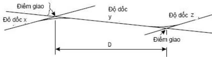
Hình A-2. Trắc dọc tim đường CHC
