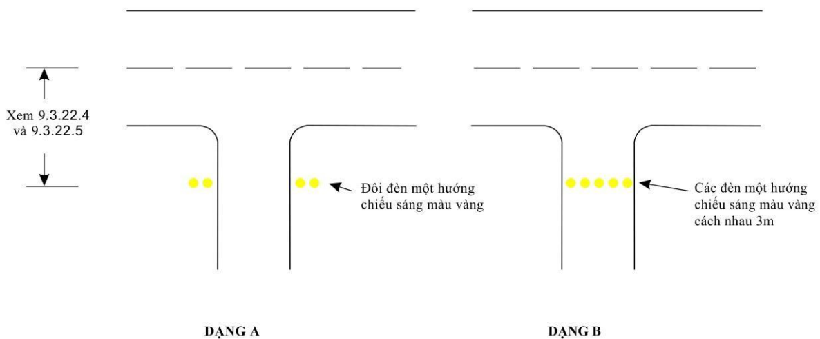
Hình 5-29. Đèn bảo vệ đường cất hạ cánh
