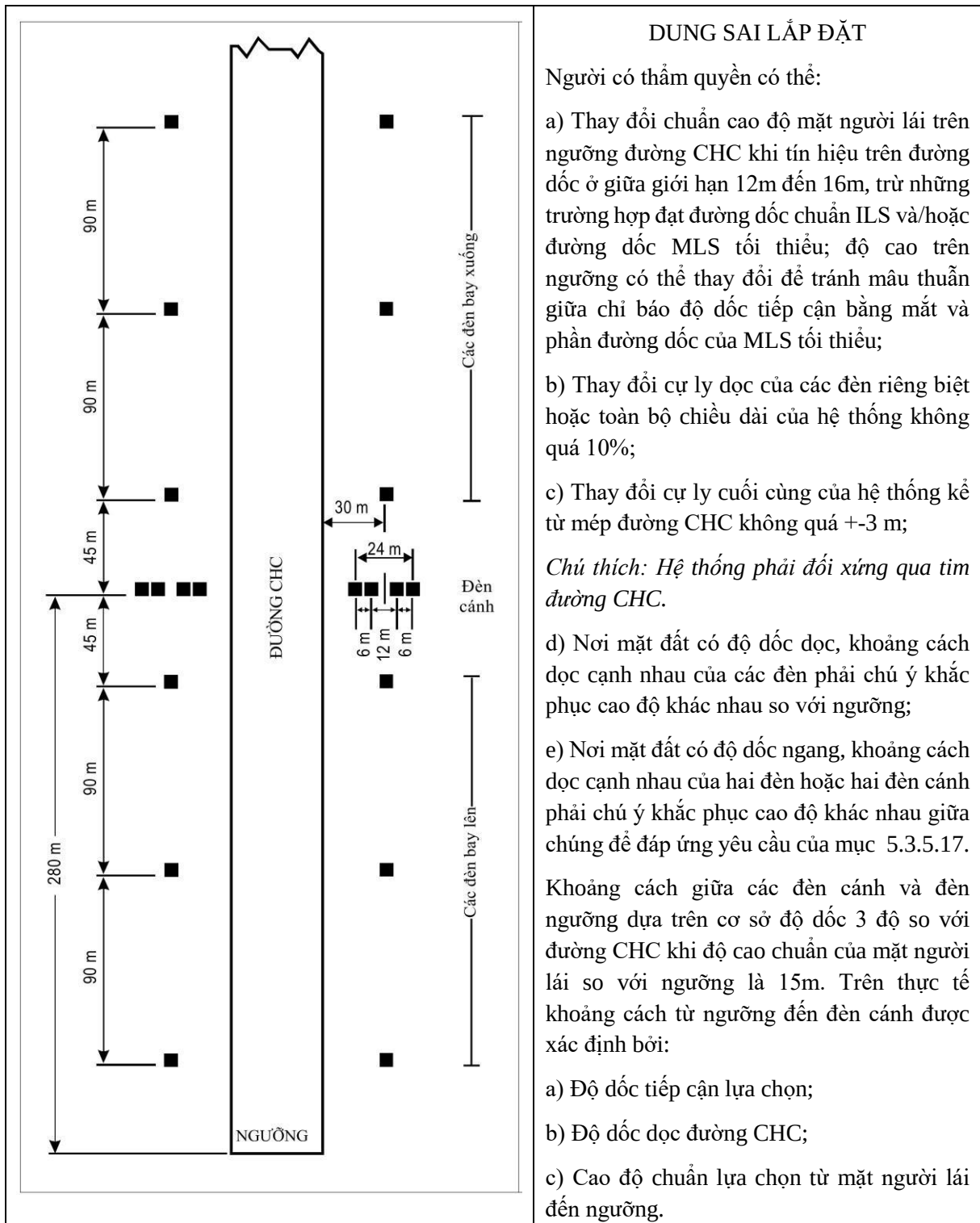
Hình 5-17. Vị trí đèn của T-VASIS
