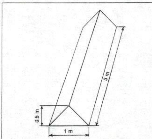
Hình 5-34. Mốc đường biên
