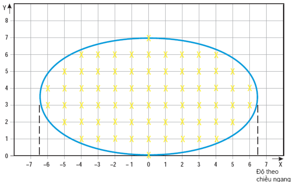
Hình A2-11. Lưới điểm trên biểu đồ dùng để tính cường độ trung bình của đèn tiếp cận và đèn đường CHC
