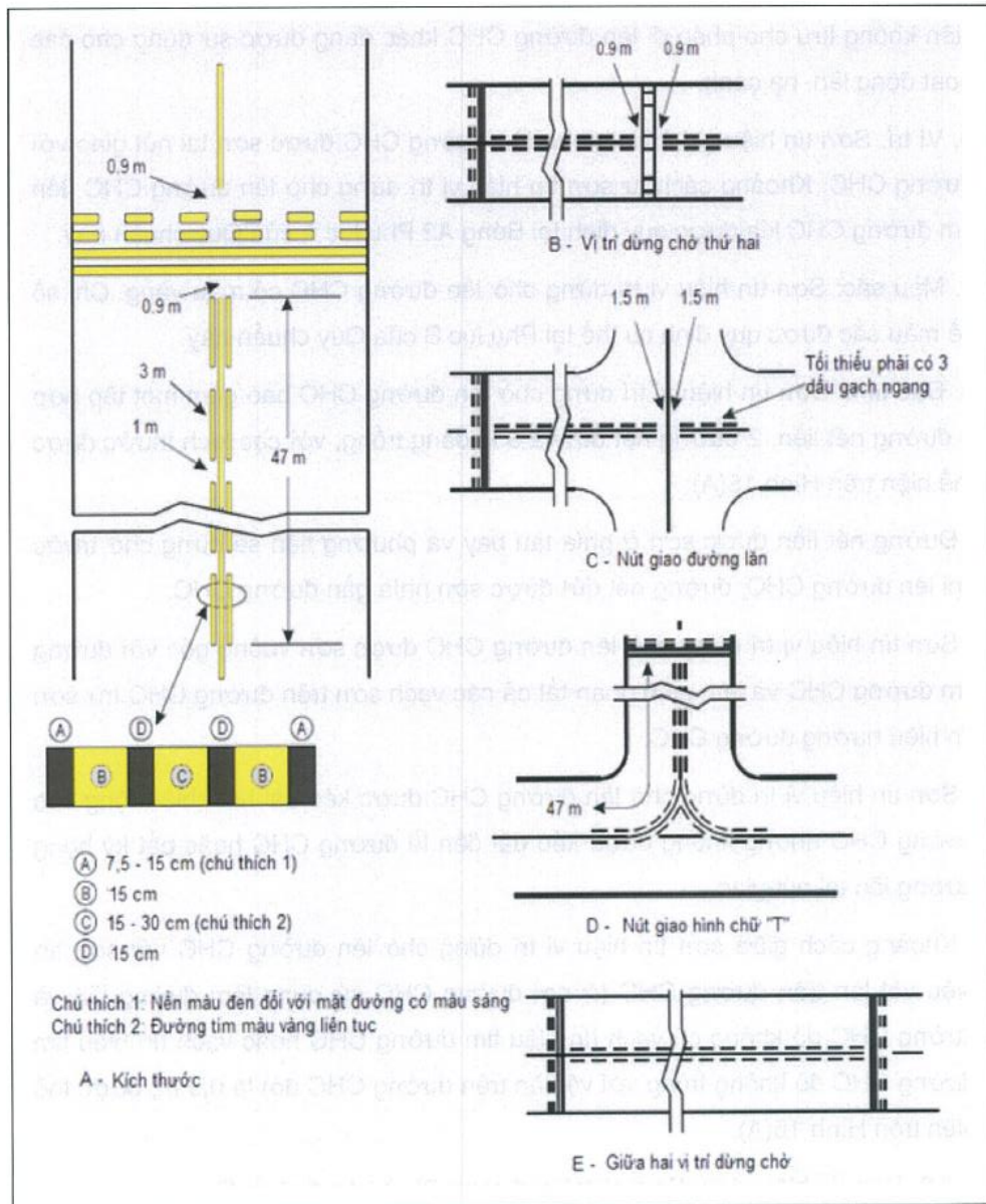
Hình 5-7. Sơn tín hiệu tăng cường cho tìm đường lẫn
