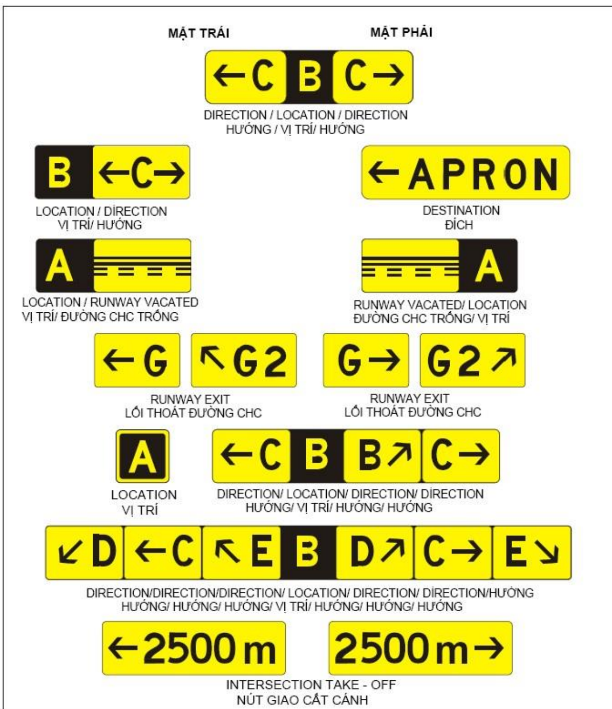
Hình 5-31. Biển báo thông tin
