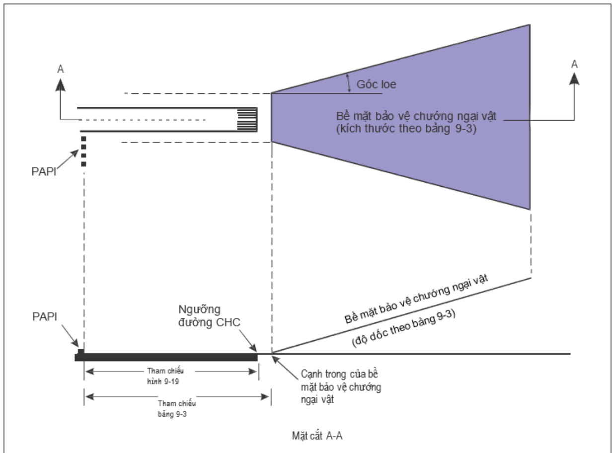
Hình 5-21. OPS cho hệ thống chỉ dẫn độ dốc tiếp cân bằng mắt
