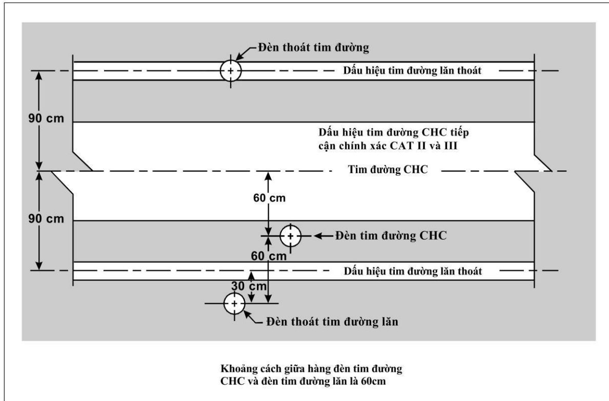
Hình 5-27. Khoảng cách giữa đèn tim đường lẫn và đường CHC
